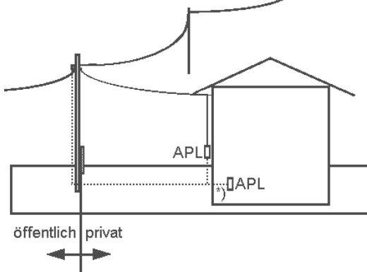
Bauweise der Hauszuführung bei oberirdischer Trassenführung auf öffentlichen Wegen
